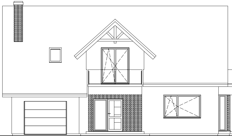
ELEWACJA FRONTOWA
