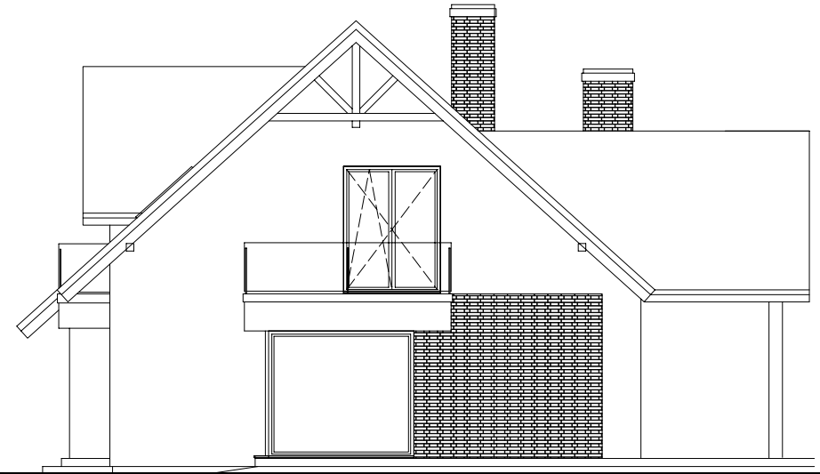
ELEWACJA BOCZNA PRAWA
